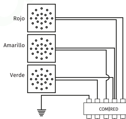
Esquema de Conexiones
